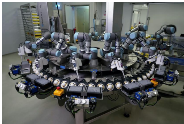
Ill. 8: Dispositif d'ovosexage de la firme Seleggt, https://www.seleggt.com/seleggt-process/
